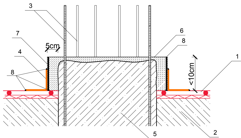
Ry. 2. Hydroizolacja głowicy pala fundamentowego - PRZEKRÓJ
