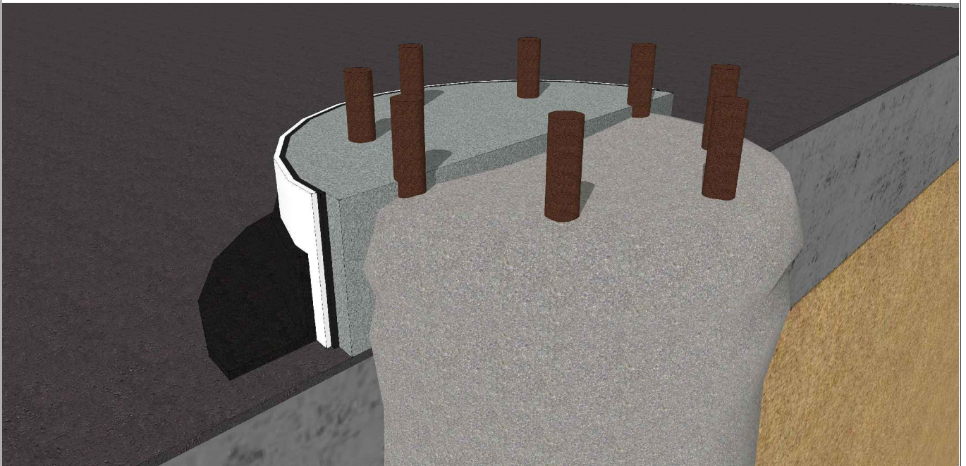
Ry. 1. Hydroizolacja głowicy pala fundamentowego - WIDOK
