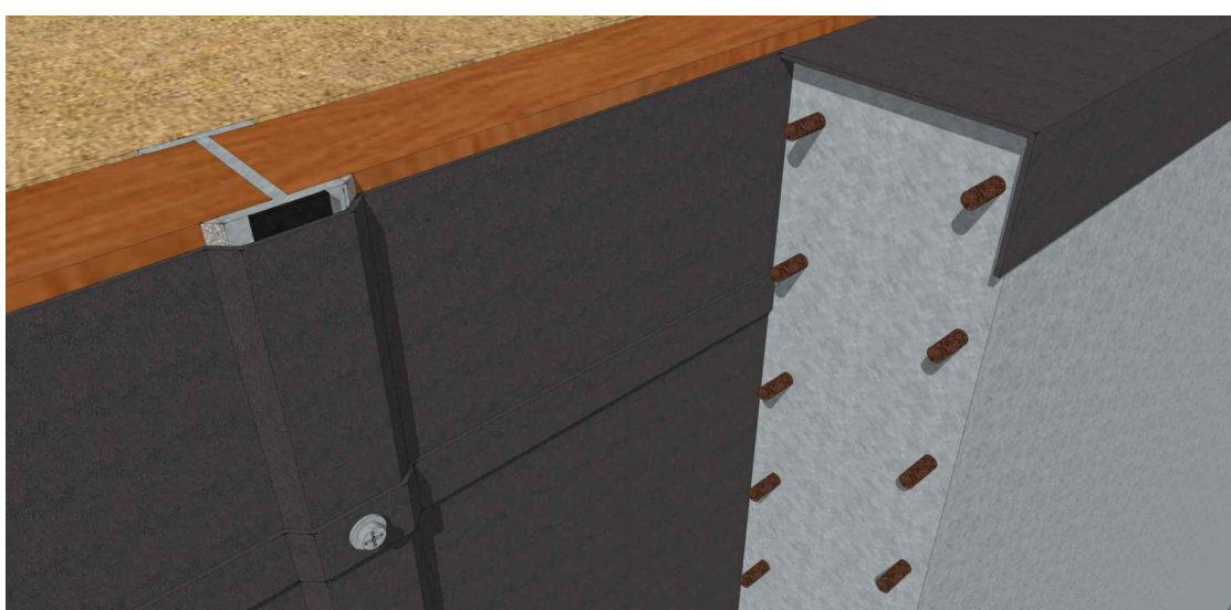
Rys. 1.2. IZOLACJA ŚCIANKI BERLIŃSKIEJ - CZĘŚĆ GÓRNA
