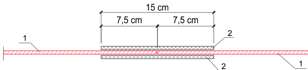
Rys. 2. POŁĄCZENIE POPRZECZNE PASÓW MEMBRAN - PRZEKRÓJ
