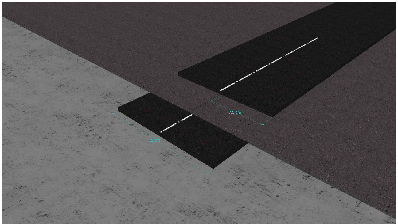
Rys. 1. POŁĄCZENIE POPRZECZNE PASÓW MEMBRAN - WIDOK
