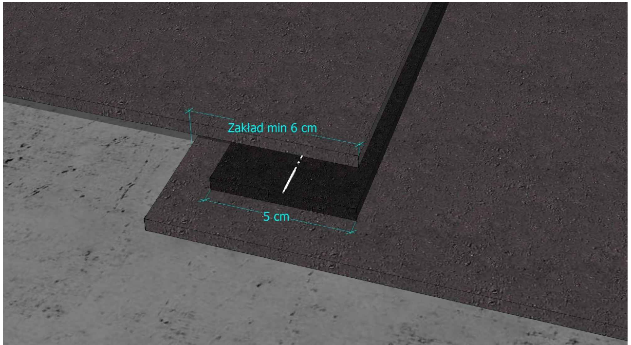
Rys. 1. POŁĄCZENIE WZDŁUŻNE PASÓW MEMBRAN - WIDOK
