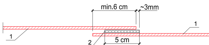
Rys. 2. POŁĄCZENIE WZDŁUŻNE PASÓW MEMBRAN - PRZEKRÓJ
