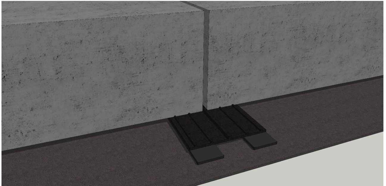
Rys. 1. USZCZELNIENIE SPOINY DYLATACYJNEJ - WIDOK
