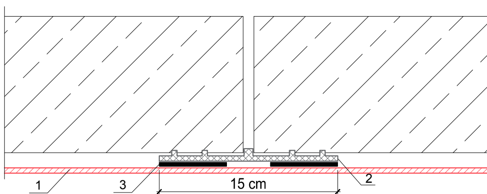
Rys. 2. USZCZELNIENIE SPOINY DYLATACYJNEJ - PRZEKRÓJ
