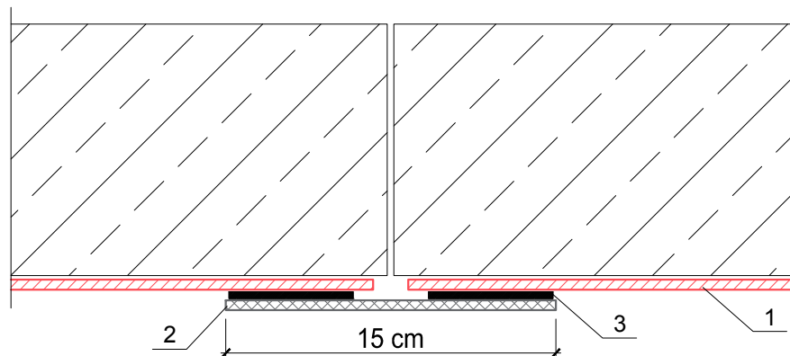
Rys. 2. USZCZELNIENIE SPOINY ROBOCZEJ - PRZEKRÓJ
